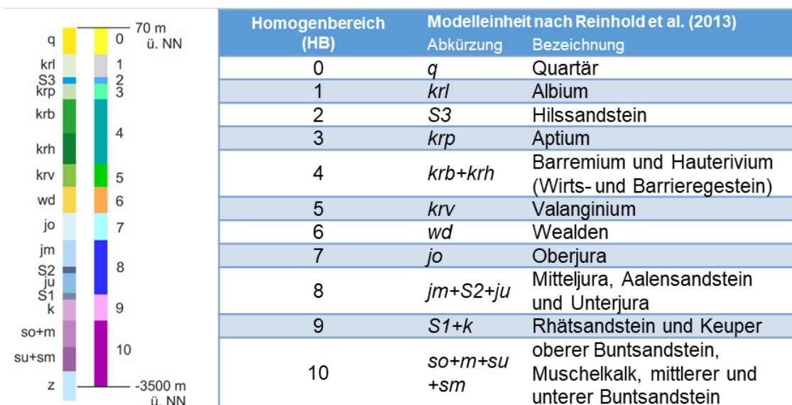
Abb. 13: Modelleinheiten: links: nach geologischen Modell; daneben: für Modellberechnungen mit den Homogenbereichen (HB) 0 bis 10
