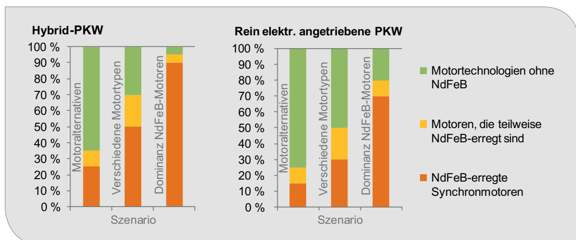
Abb. 4.3: Für 2035 geschätzte Anteile von Technologien für Traktionsmotoren, welche vollständig, teilweise oder nicht auf einer permanentmagnetischen Erregung durch NdFeB-Magnete beruhen (Quelle: eigene Darstellung)
