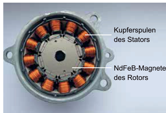
Abb. 4.105: Lenkungsmotor eines PKW (Quelle: eigenes Werk)
